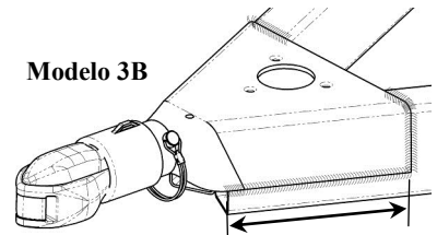
Traslapeo mínimo de la horquilla - 6.5"
