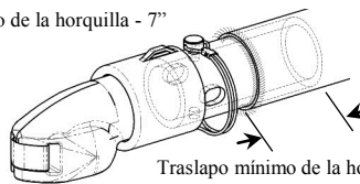
Traslapeo mínimo de la horquilla - 2.5" (La horquilla puede ajustarse sobre o dentro del acoplador)
