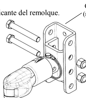
Pernos provistos
